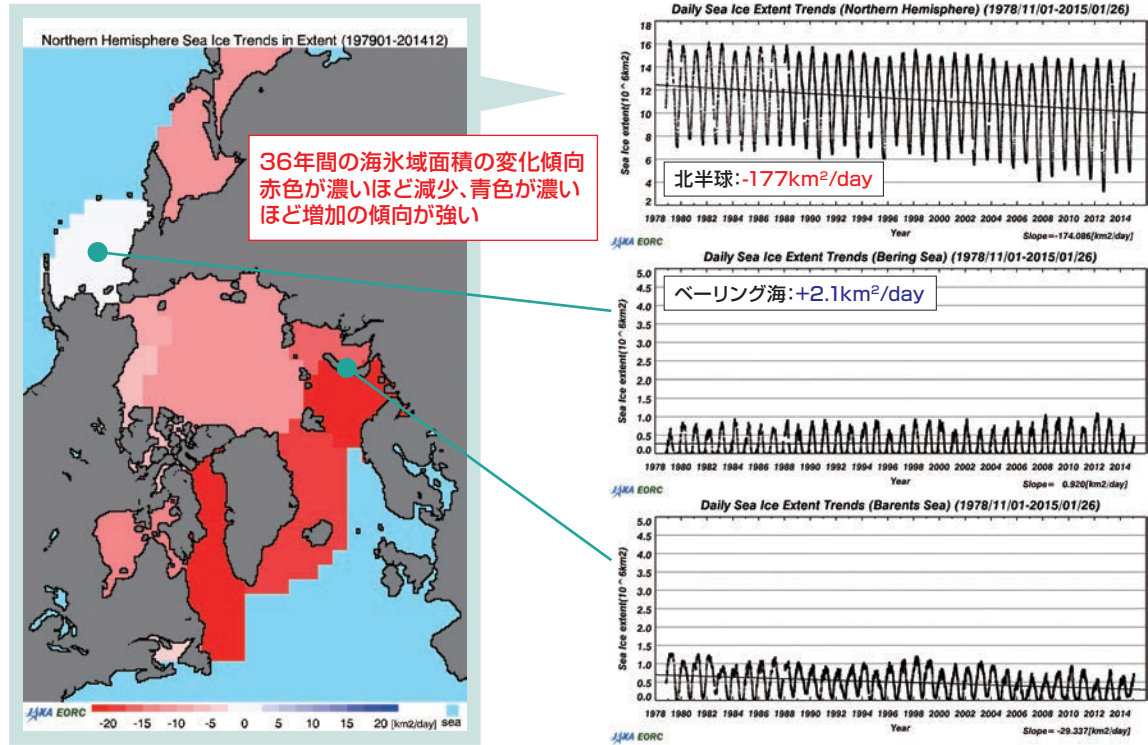
海域別の海水域面積の長期トレンド(1978-2014年)
