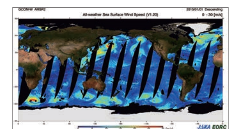
全天候海上風速(研究プロジェクト)
