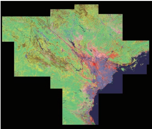
高解像度土地利用土地被覆図ベトナム北部版 Version 16.09
