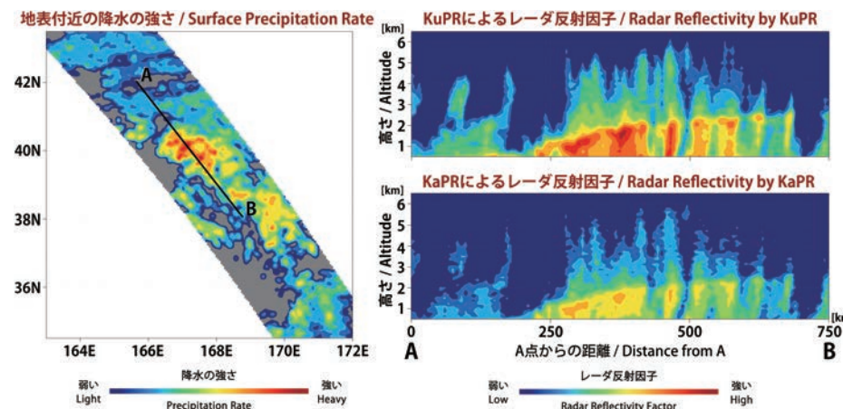
DPRによる降水の三次元分布(JAXA/NASA)
