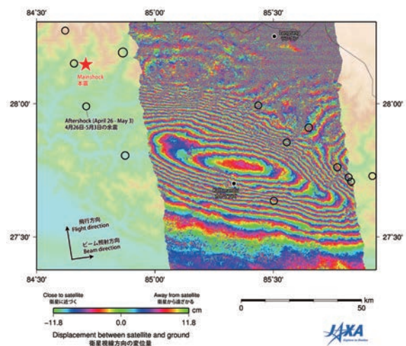
ネパール地震前後(前: 2015年2月21日、後: 2015年5月2日)に取得されたPALSAR-2データによる干渉画像
