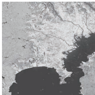
東京周辺(SARモザイク、HH偏波)
