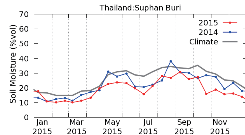
タイ王国スファンブリ県における土壌水分量の時間変化
